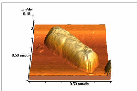
Slika 2 - Pojedinačna ćelija At. ferrooxidans soj B 4 (3D prikaz topografije, površina snimanja 2,5 µm x 2,5 µm).
